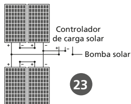
PANEL SOLAR: 4 x 265W
