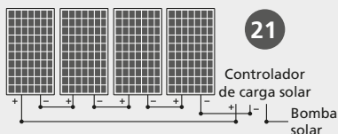
PANEL SOLAR: 4 x 265W
